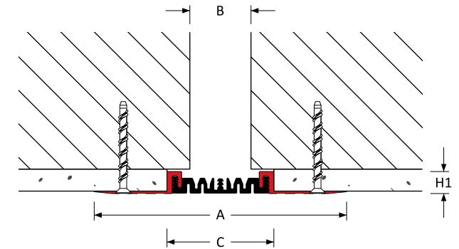
Maxatec 150 : A07
