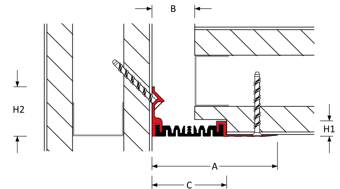
Maxatec 150 : A09
